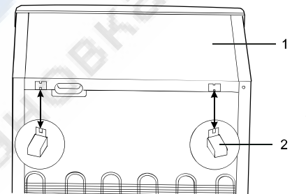
Рисунок Б.2 - Схема кріплення упорів до кришки Рисунок Б.2 - Схема крепления упоров к крышке Şəkil B.2 - Dayaqların qarağa bərkidilmə sxemi Б.2-сурет - სახურავზე საყრდენების დამაგრების სქემა B.2-сурет - Tipeyişti қақпаққа бекіту схемасы Figura B.2 – Schema fixării de sarac a opritorului B.2-rasm: Tirgakların ustki qismga oʻrnatish chizmasi.
