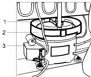
Рисунок Б.4 - Схема відведення талої води з холодної камери Рисунок Б.4 - Схема отвода талой воды из холодильной камеры ნახაზი Б.4 - სამაცივრე კამერიდან გაღობილი წყლის გადმოსვლის სქემა Şəkil B. 4 - Soyuducu kameradan erimiş suyun axma sxemi Б.4-сурет - Тоңазытқыш камерадан еріген судың ағу сызбанұсқасы Figura B.4 - Schema scurgerii apei dezghețate din camera frigorifică B.4-rasm: Muz erishidan hosil bo'lgan suvni sovutish kamerasidan chiqarib tashlash chizmasi
